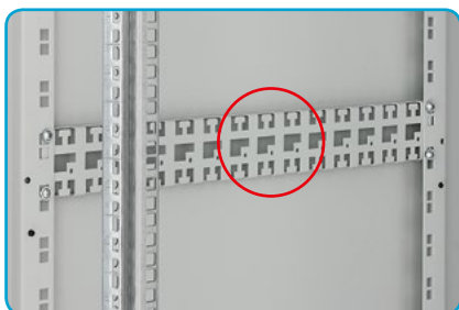
■ RAC-VP-D5x-X1 Horizontale Kabelführungsstrebe (optionales Zubehör)
