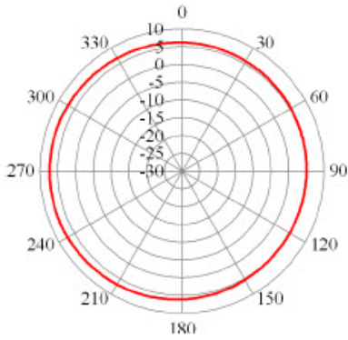
— 868MHz Horizontal
