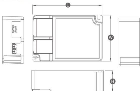
Dimension(unit:mm)
