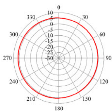
— 868MHz Horizontal
