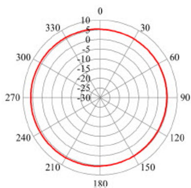
— 868MHz Horizontal
