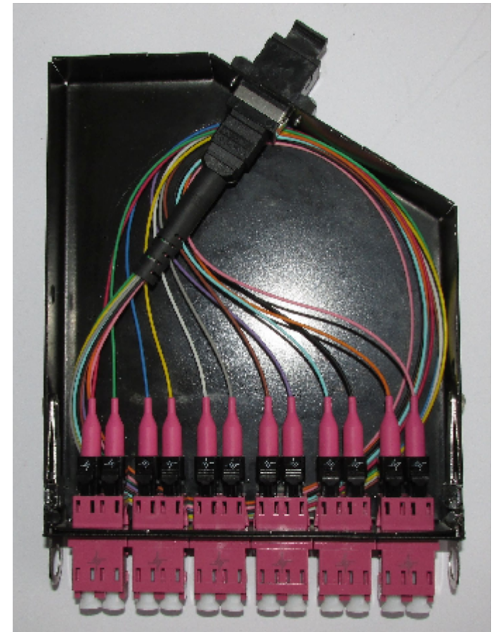
Beispiel für Einbau / Example of mounting FanOut-Kit
