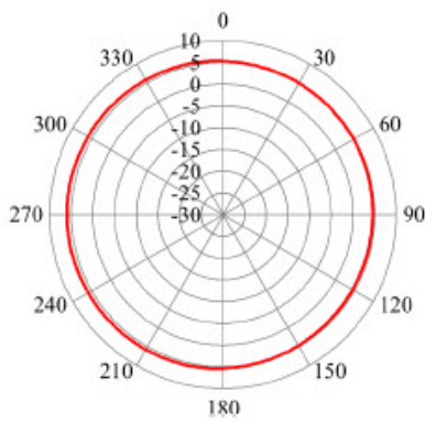
— 868MHz Horizontal
