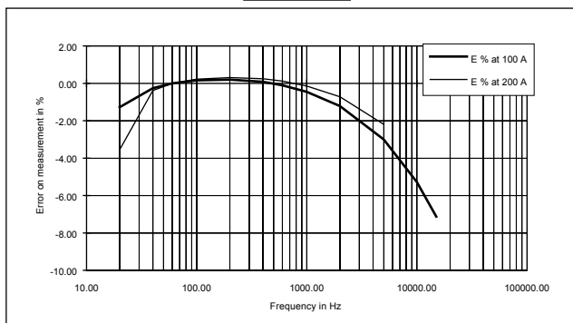
200 A calibre
