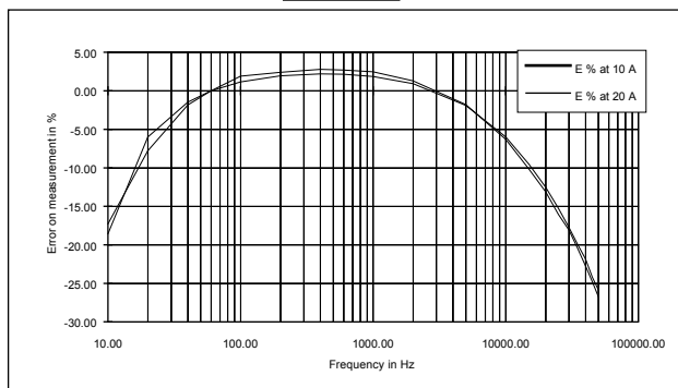
20 A calibre
